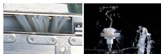
ウォーターモータ採用のターボジェットブラシ
